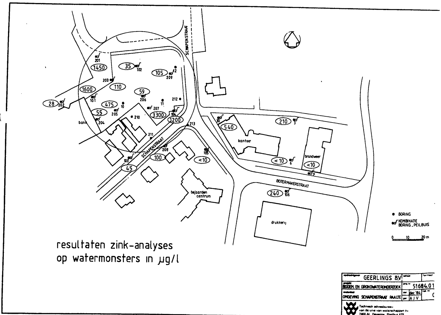
Figuur 3. Verspreiding van zink in het grondwater (fase 1 + 2)
