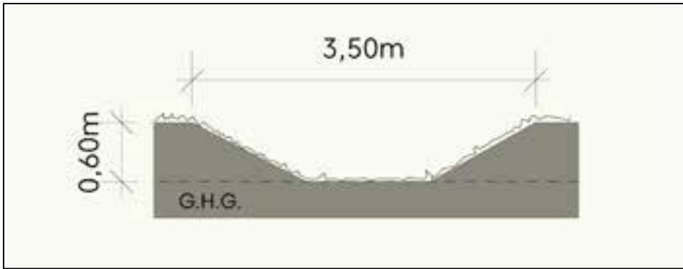
Abbeelding 7.1 Profiel nieuw te graven sloot (Bron: de Erfontwikkelaar)
