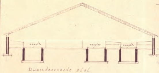
Dwarsdoorsnede stal
