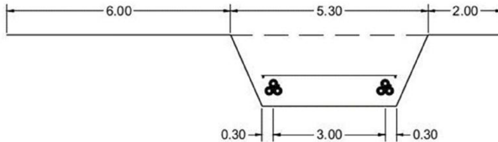
Afbeelding 4. Principedoorsnede van het kabeltracé (bron: TenneT TSO B.V.)
