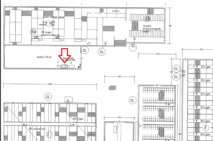
figuur 2: situering bovengrondse tank periode 2003
